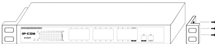
G1216T/G1224T 安装 L 型支架示意图 (以 G1224T 为例)
