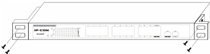
G1216T/G1224T 机架固定示意图 (以 G1224T 为例)
